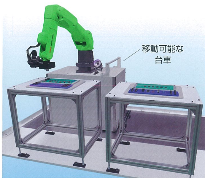
電子基板組立
