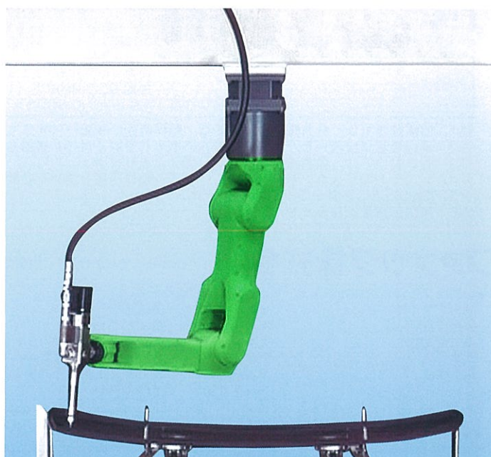
フロントガラスへの接着剤塗布（天吊り設置）
